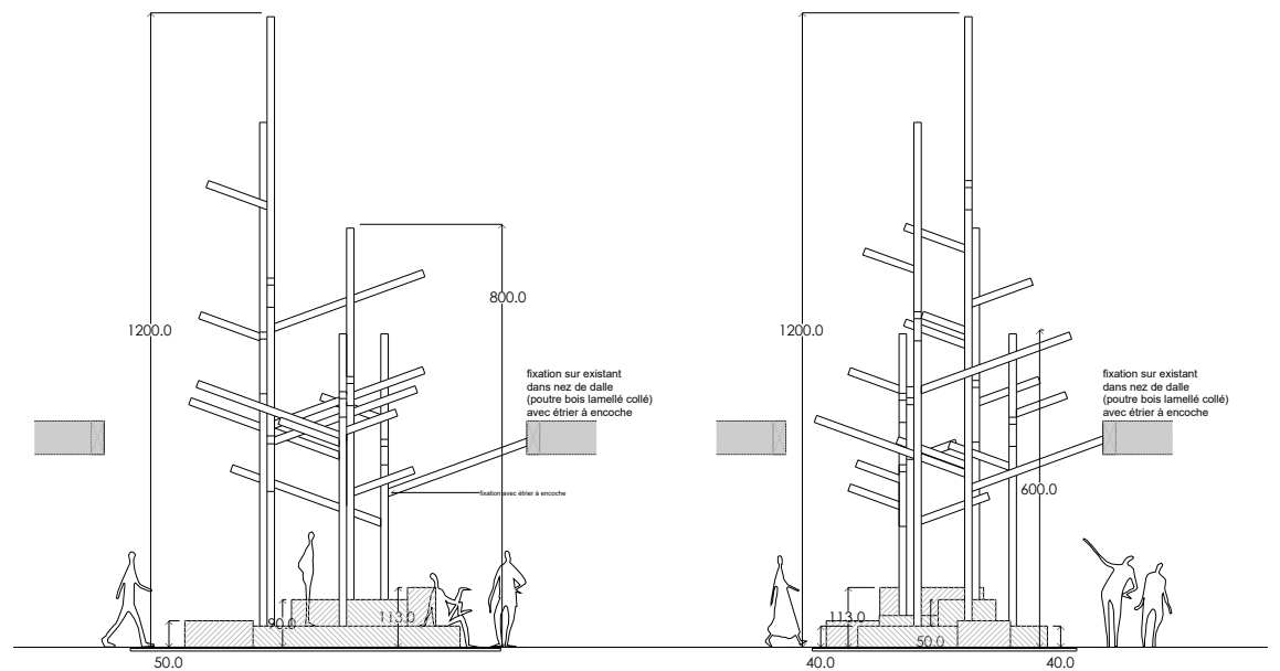
Elevations 1/50 dimensions en cm
